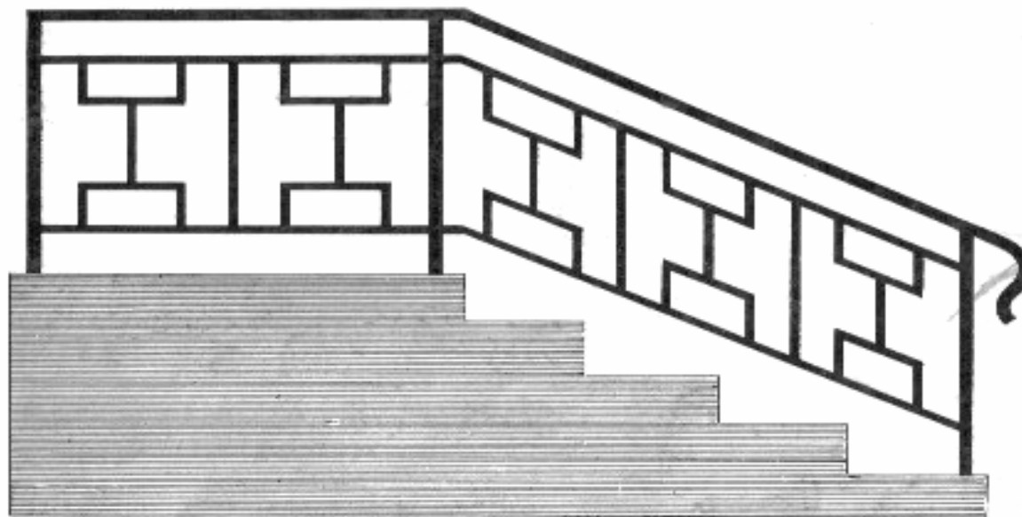
Trappräck modell 10
